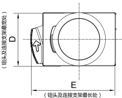
图 4 LA42(V) 系列按钮外形图
