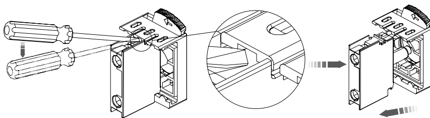
正确拆卸
