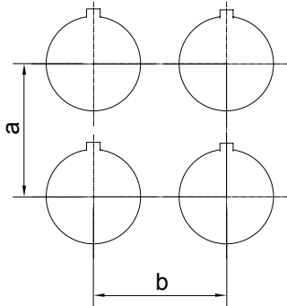
图 5 LA42(V) 系列按钮安装中心距尺寸
