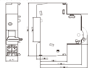
外形及安装尺寸
