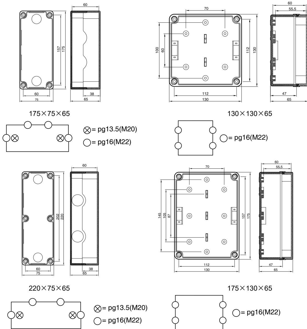
外型尺寸图·敲落孔位置图
