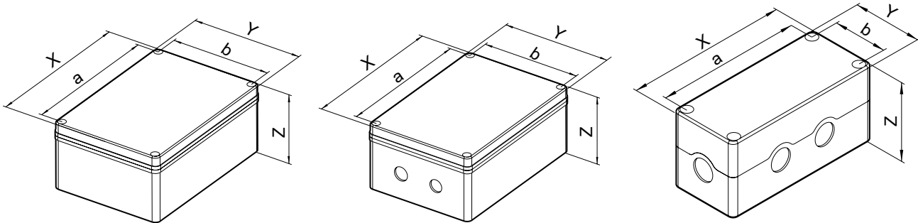
085系列无敲落孔 085系列有敲落孔 085系列有敲落孔
