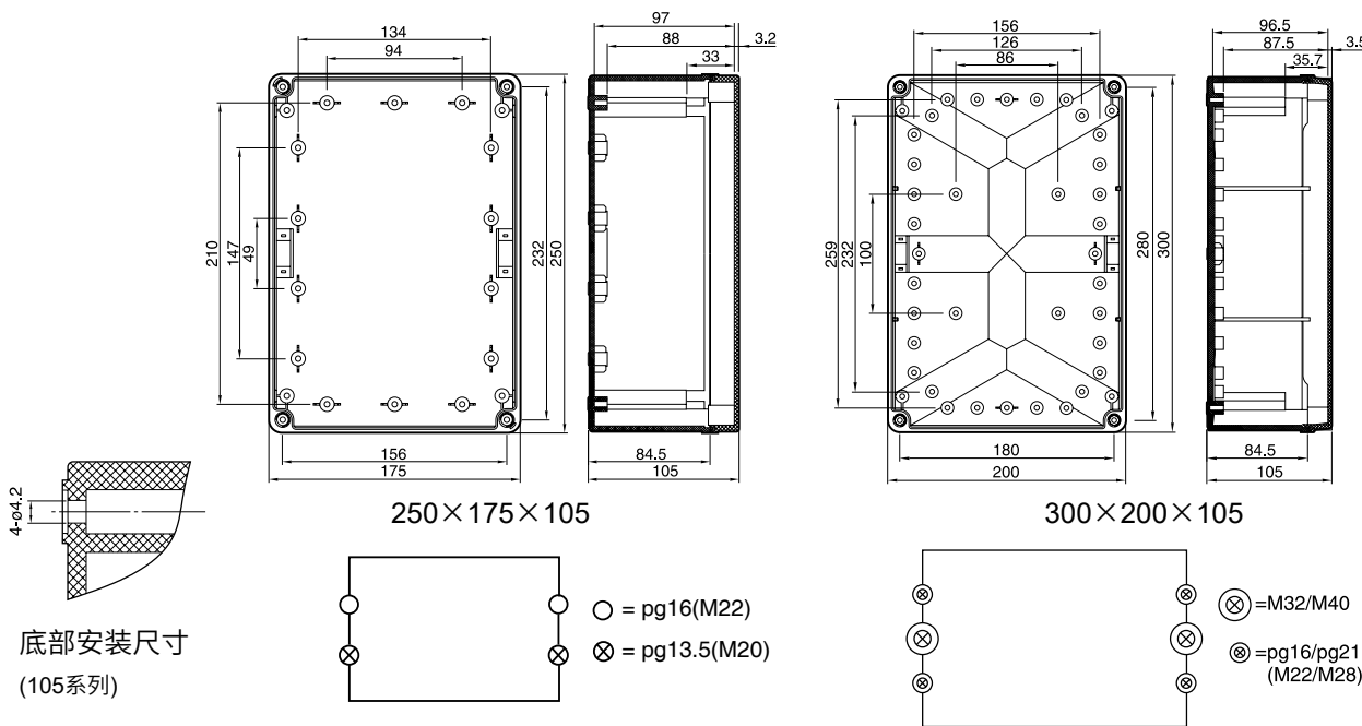
外型尺寸图·敲落孔位置图
