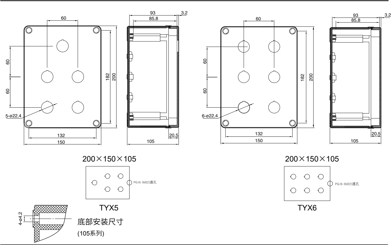
外型尺寸图·敲落孔位置图
