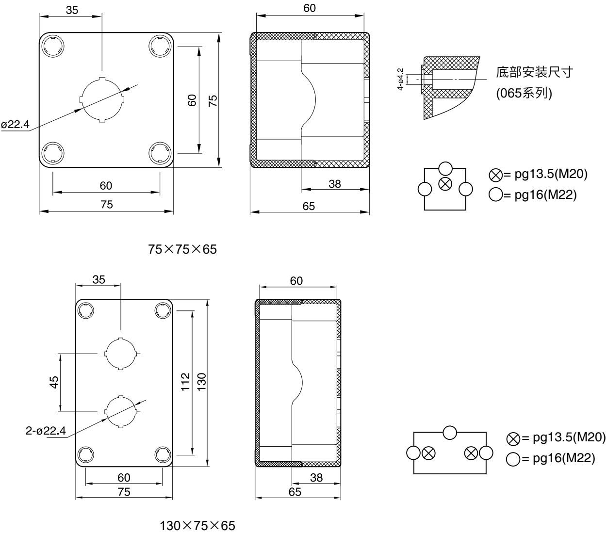
外型尺寸图·敲落孔位置图
