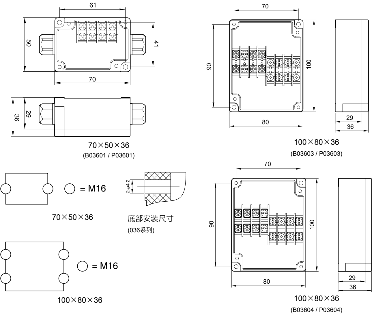
外型尺寸图·敲落孔位置图
