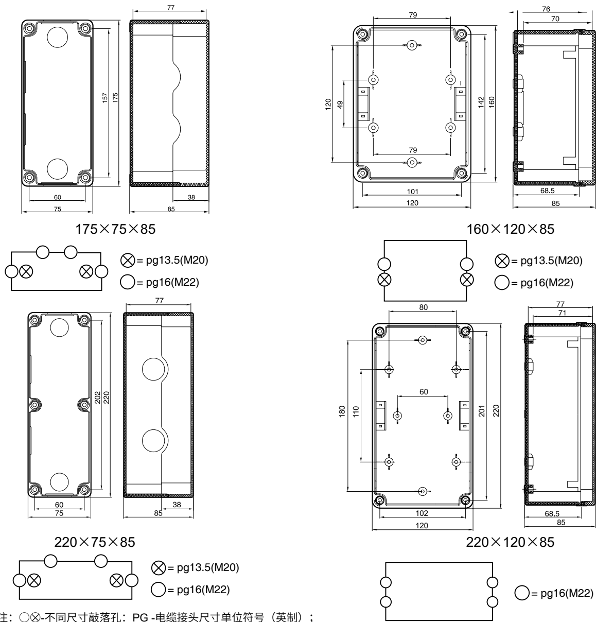
外型尺寸图·敲落孔位置图
