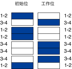
图1.二位置
