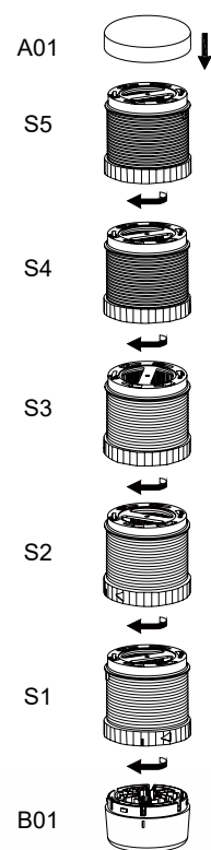
安装图
