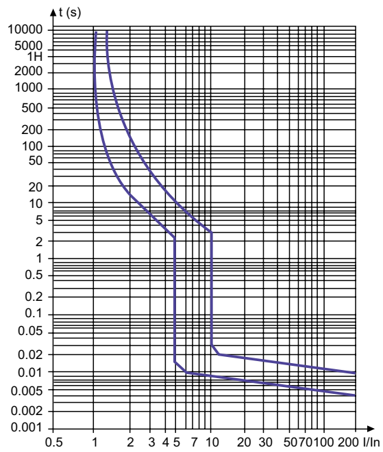
C 曲线
