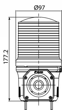
直接安装尺寸
