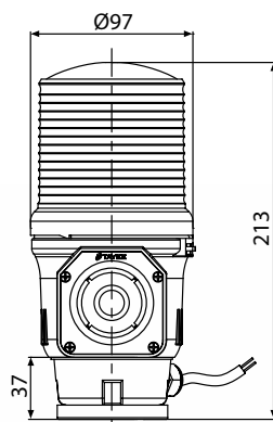
竖直安装（配S-2）
