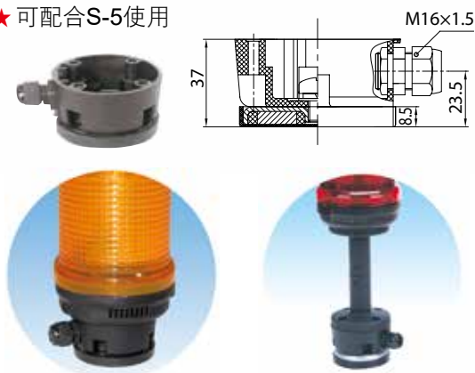
侧向安装底座(内走线) C-5
