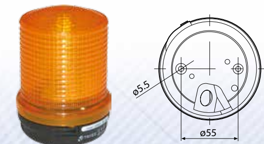
直接安装(内走线)
