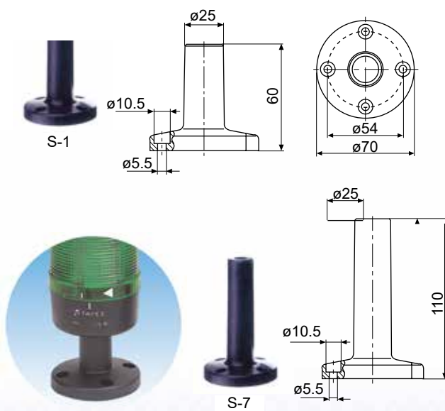
竖直安装底座(内走线) S-1, S-7
