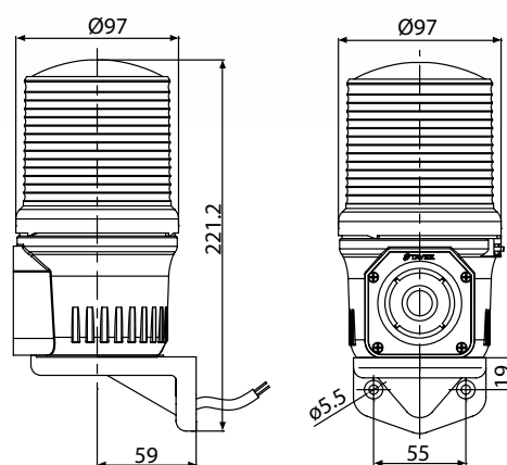
侧向安装尺寸（配C-5）
