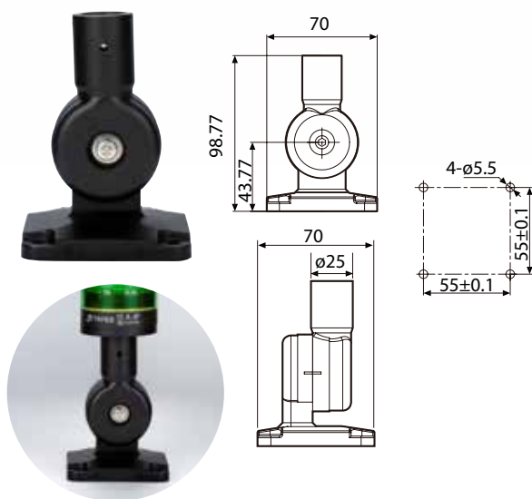
可折叠安装底座（内走线） SC-3B
