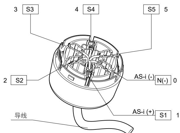
导电座接线图
