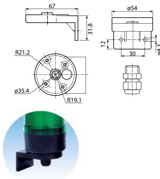
侧向安装底座(外走线) C-6
