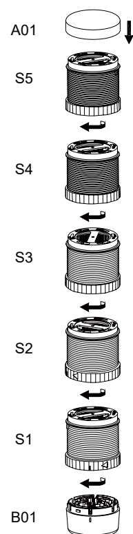
安装图
