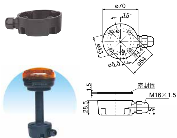
直接安装(内走线)
