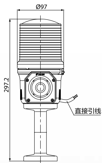
竖直安装尺寸（配S-5）
